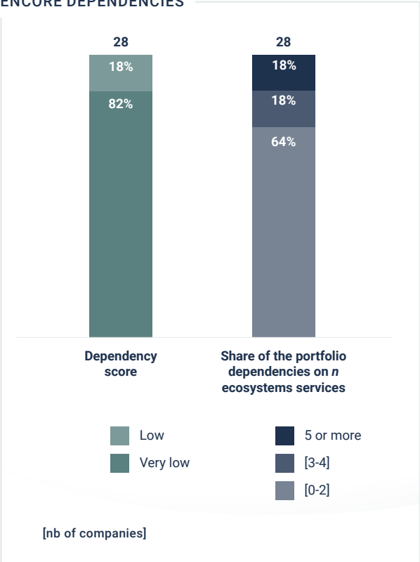
ENCORE DEPENDENCIES
