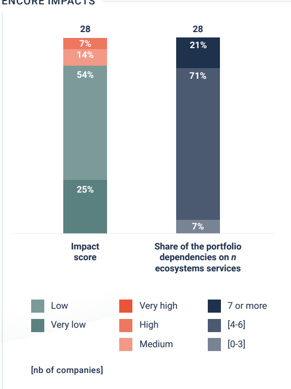
ENCORE IMPACTS
