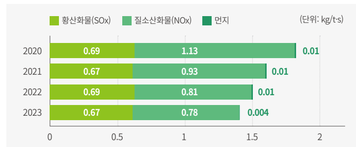
조강 1톤당 배출량 연간 추이
