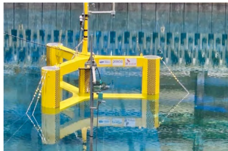
2023년 9월 26일 대전 선박해양플랜트연구소에서 열린 수조실험에 공개된 ‘K-부유체’ 36분의 1 축소 모델(폭 약 2m, 높이 약 1m)
